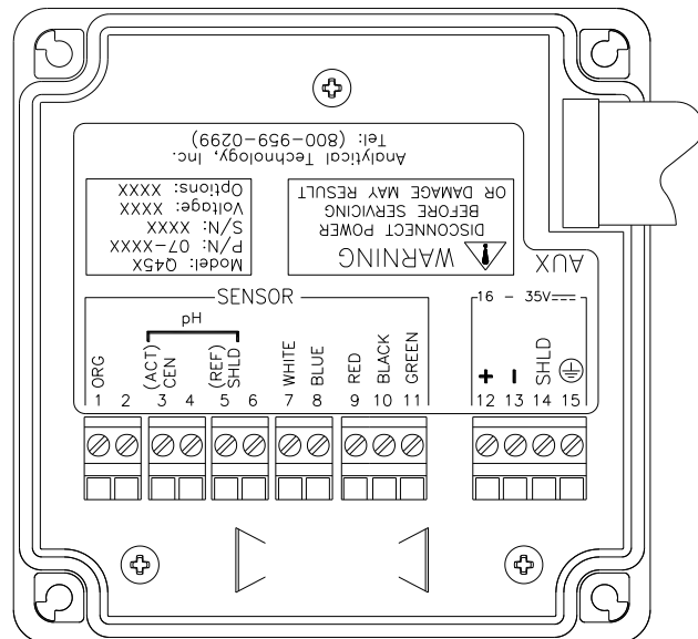
O3 SENSOR WIRING
